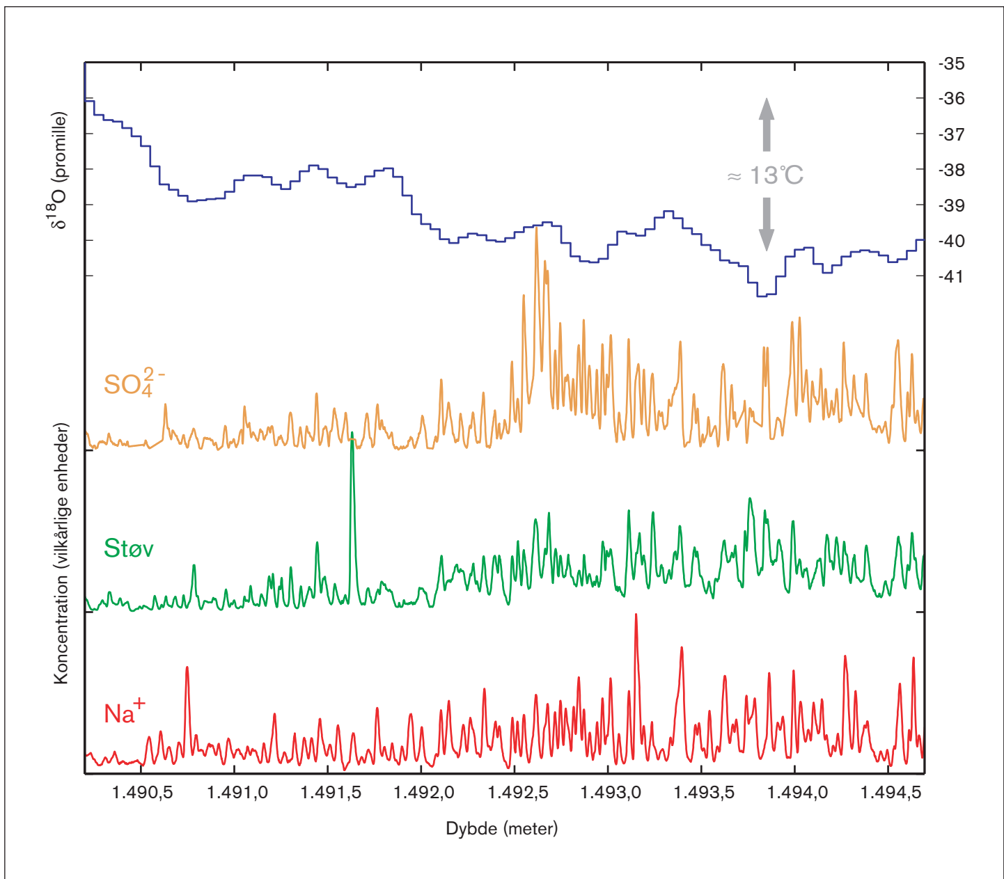
5. NordGRIP-iskernens indhold af \text{Na}^+ -ioner, \text{SO}_4^{2-} -ioner og støv samt isens isotopsammensætning (boks 2). Højre del af figuren er Yngre Dryas' afslutning, og venstre er Holocæns begyndelse. Årlagstykkelsen og indholdet af urenheder ændres ganske brat, mens isotopsammensætningen – og dermed temperaturen – ændres mere gradvis.
