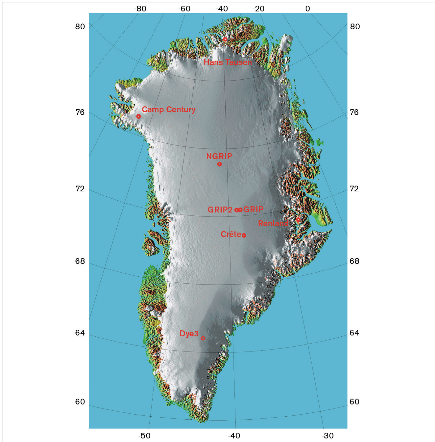
2. Placeringen af de borelokalteter på Indlandsisen hvor der er boret iskerner ned til bunden, de såkaldte dybe iskerner. NordGRIP er markeret som NGRIP på kortet. (Kilde: Kort- & Matrikelstyrelsen)
